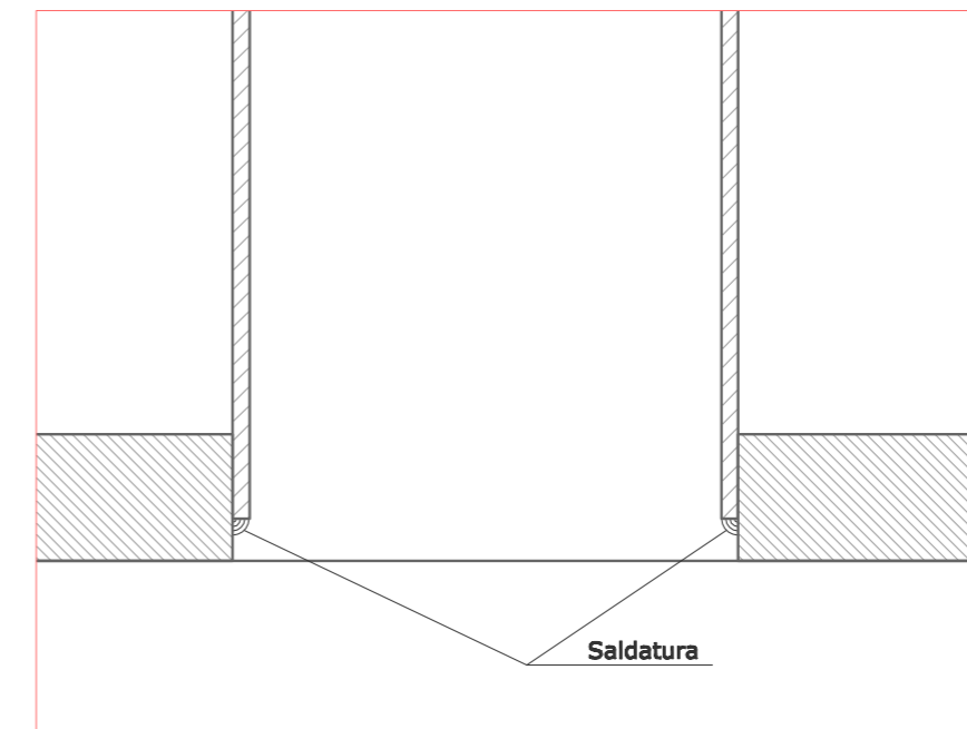
Dettaglio saldatura tra basamento e elemento tubolare Scala 1:1
